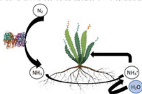
图 1 固氮原理
